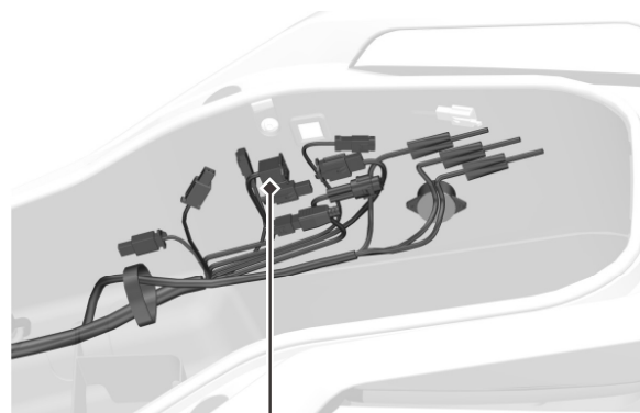
Conector para el inmovilizador
